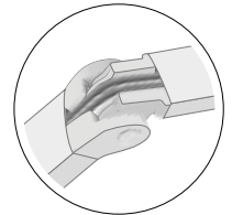
Articulation du bras à double câble gainé Testés à 20 000 cycles
